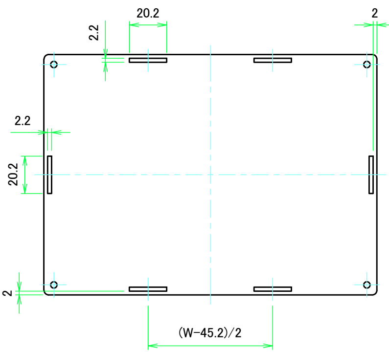
上カバー裏面 / Top cover Backside
