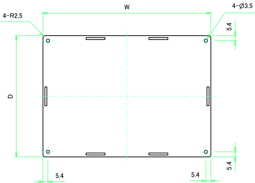
上カバー表面 / Top cover Frontside
